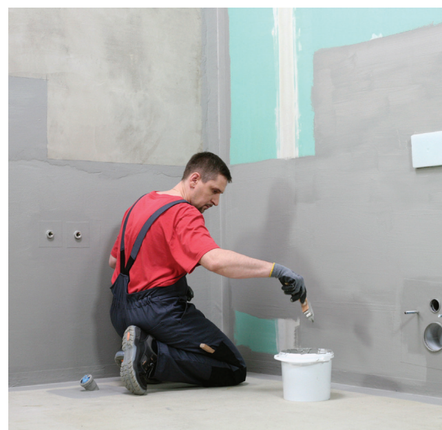
Application des première et seconde couches d'isolant à l'aide d'un pinceau.
